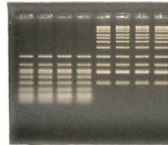
TBE バッファ用 1.5% アガロースゲル 50 V、60 分泳動 EtBr 染色 30 分
