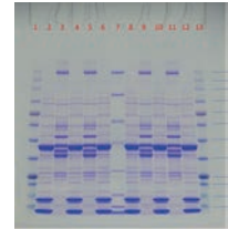
7.5~15% グラジエント PAGE-中性ゲル 300 V、33 分泳動
