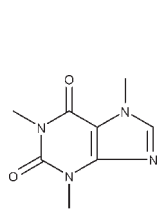
Caffeine
